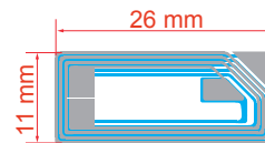
天线图 (Antenna)
